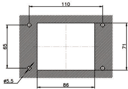
32B不封口底座安装 面板开孔尺寸
