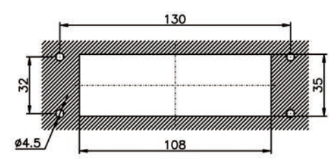
24B底座 面板开孔尺寸
