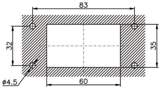
10B底座 面板开孔尺寸
