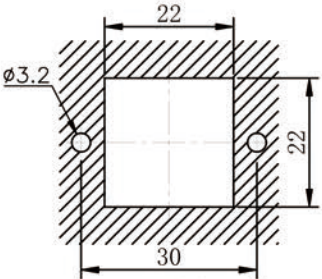
3A底座 面板开孔尺寸
