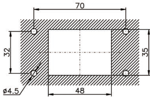
6B底座 面板开孔尺寸
